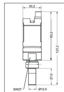
Abmessung FO 510
